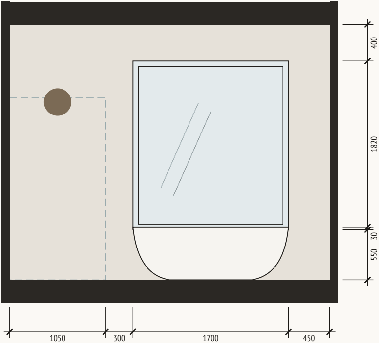
Развёртка В. Ванная, стена с окном
