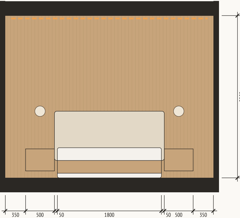
Развёртка Д. Спальня, стена за кроватью
