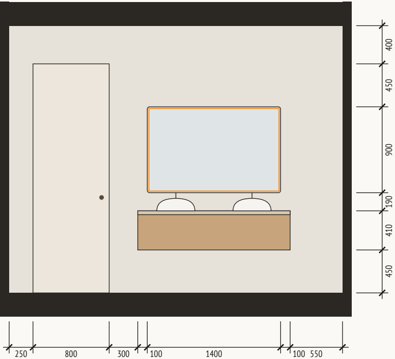
Развёртка Г. Ванная, стена с умывальниками
